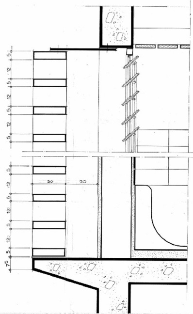
ΤΟΜΗ CLAUSTRA ΚΑΙΜΑΞ 1:5
