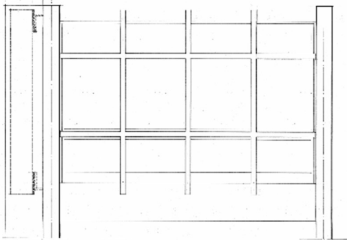
ΟΨΗ ΚΑ 1:20
