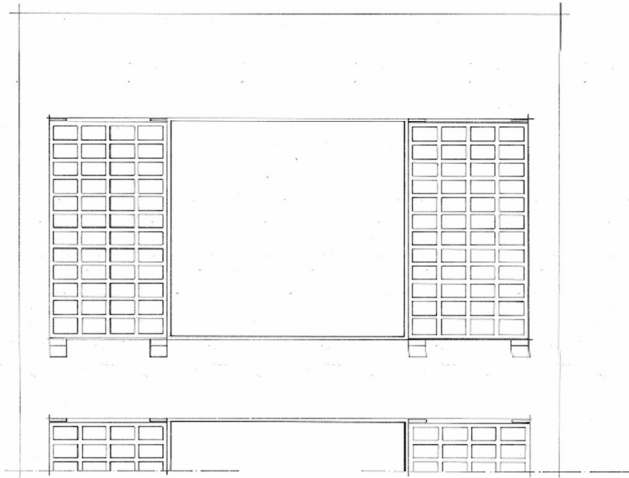
ΟΨΗ CLAUSTRA ΚΑΙΜΑΞ 1:20
