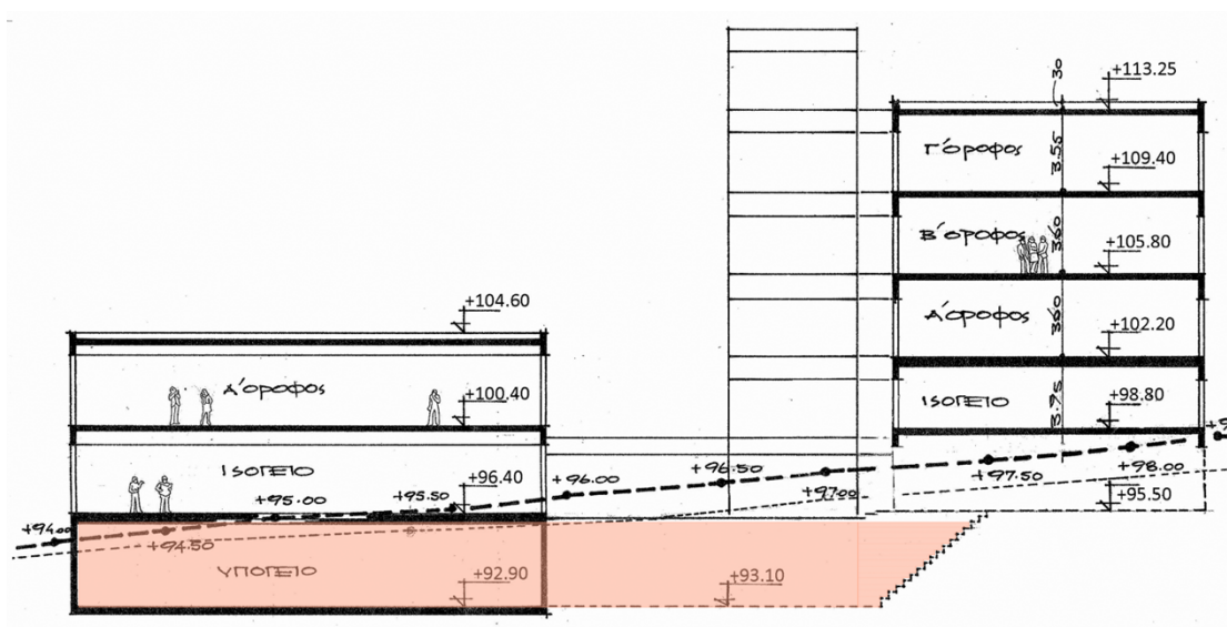
3. Ενδεικτική Τομή
