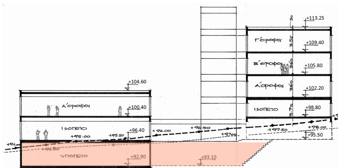
3. Ενδεικτική Τομή
