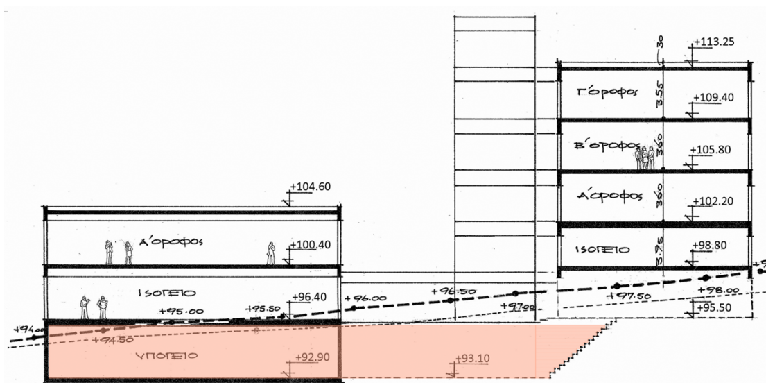
3. Ενδεικτική Τομή
