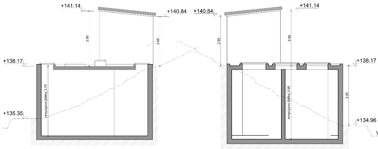
ΤΟΜΗ Γ-Γ (ΒΟΡΕΙΑ ΟΨΗ)
