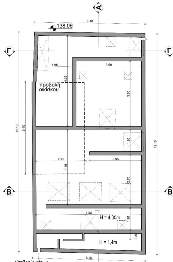
ΚΑΤΟΨΗ ΔΕΞΑΜΕΝΩΝ
