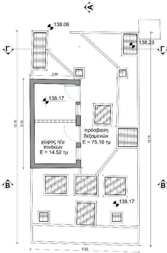
ΚΑΤΟΨΗ ΑΝΩΔΟΜΗΣ
