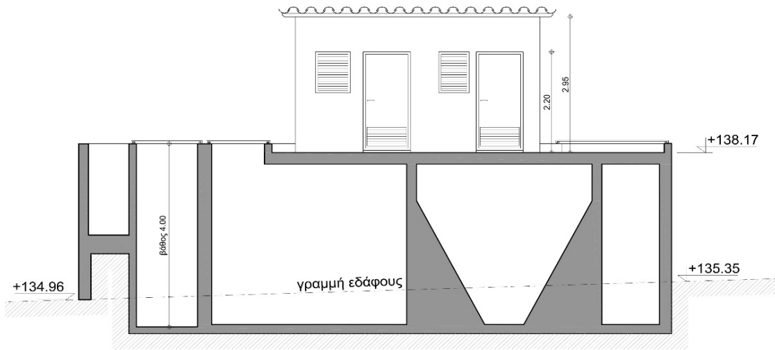
ΤΟΜΗ Α-Α (ΑΝΑΤΟΛΙΚΗ ΟΨΗ)
