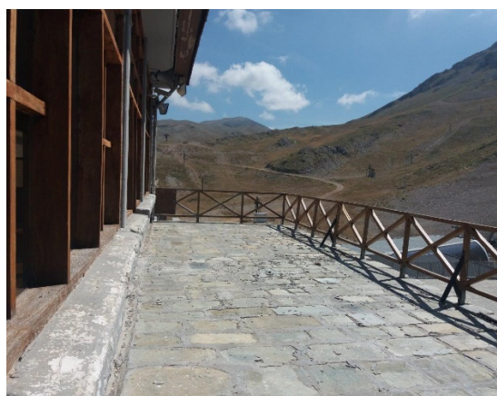
24.Τμήμα του εξώστη όπου φαίνονται ατυχείς προηγούμενες επεμβάσεις αρμολογήματος των πλακών Καρύστου.
