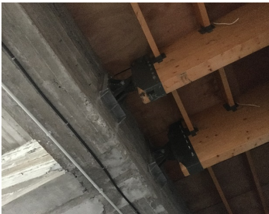
5. Έδραση ξύλινων δοκών επί δοκού από οπλισμένο σκυρόδεμα.
